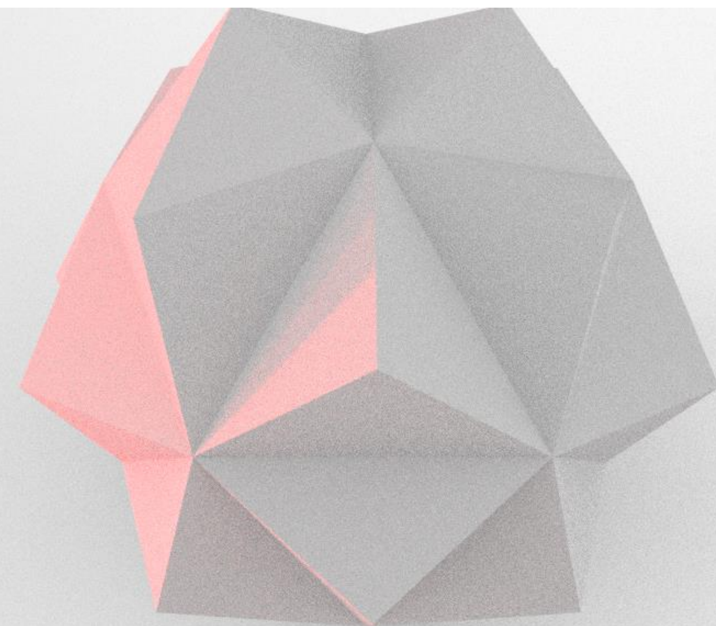
Dual do Dodecaedro Truncado
